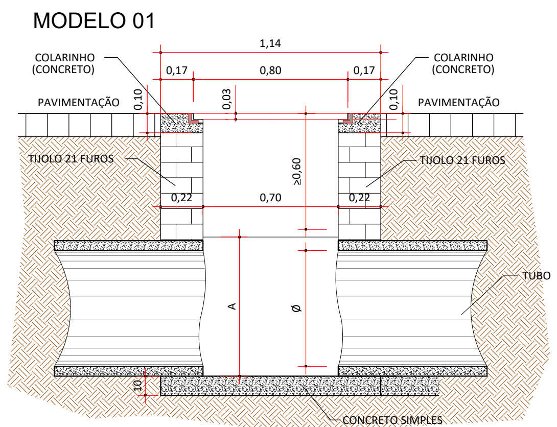
CORTE LONGITUDINAL (A A) ESC.: 1:20
