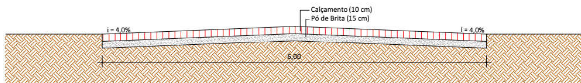
SEÇÃO TIPO
