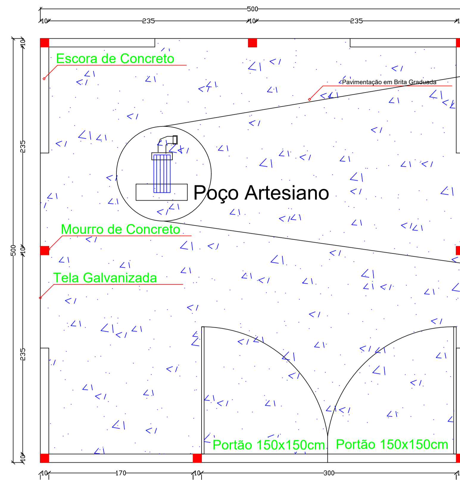
Planta Baixa da Cerca Proteção do Poço Artesiano escala 1:25
