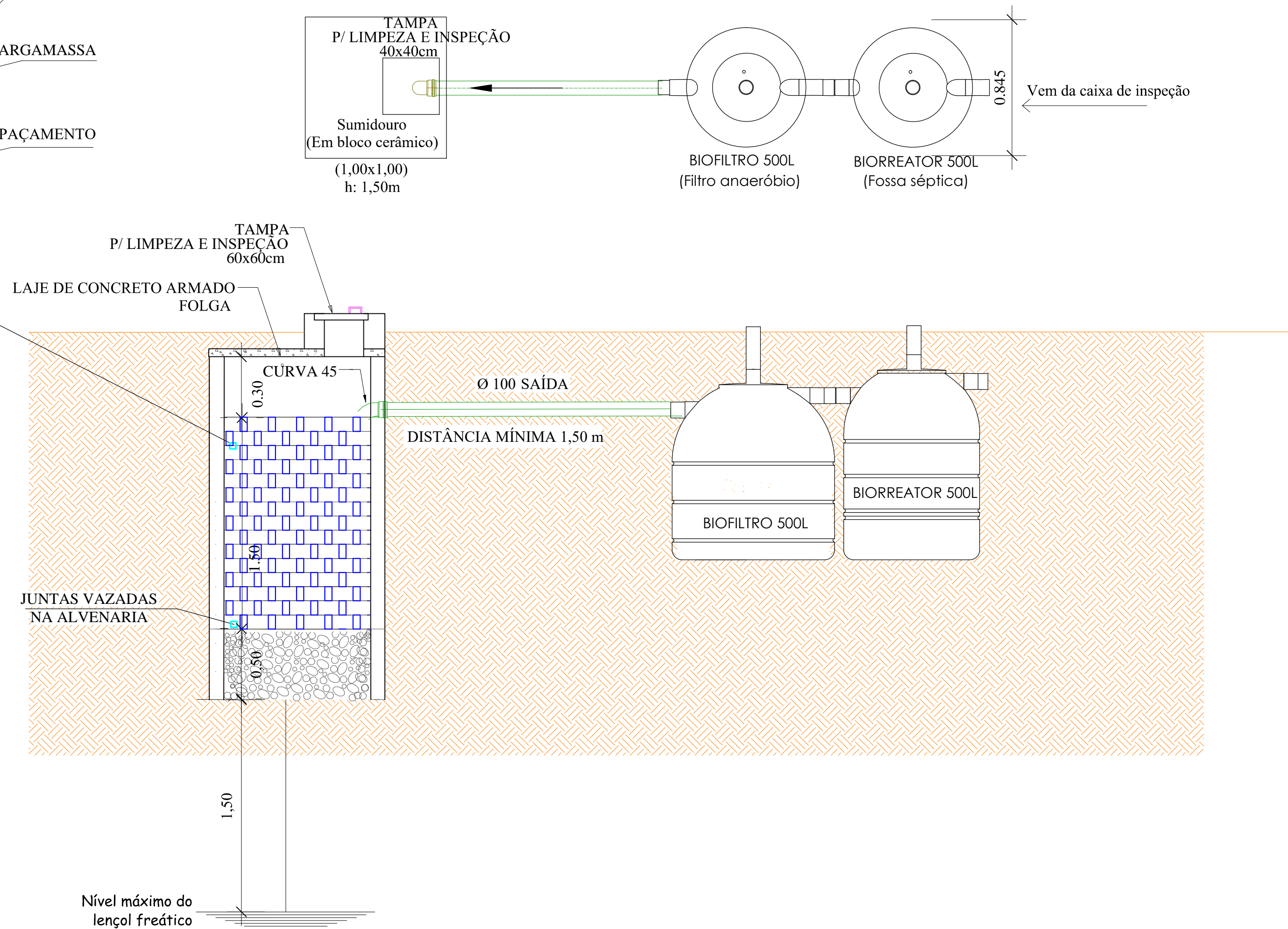
DETALHE DA ALVENARIA VAZADA
