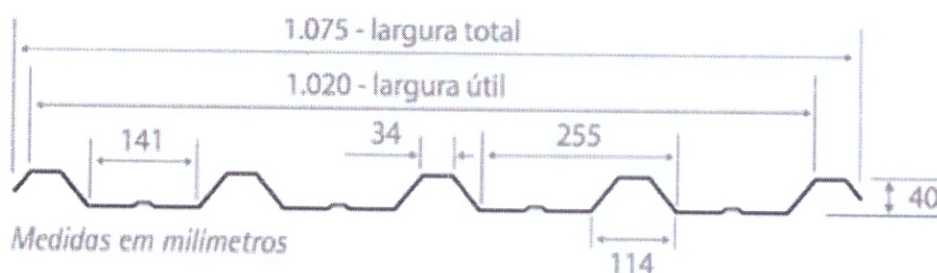
DESENHO TÉCNICO | TRAPÉZIO 40x1020
