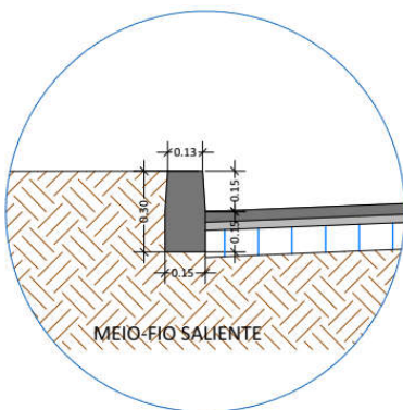
DETALHE 01 ESC.: 1 : 20
