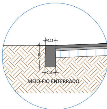
DETALHE 02 ESC.: 1 : 20
