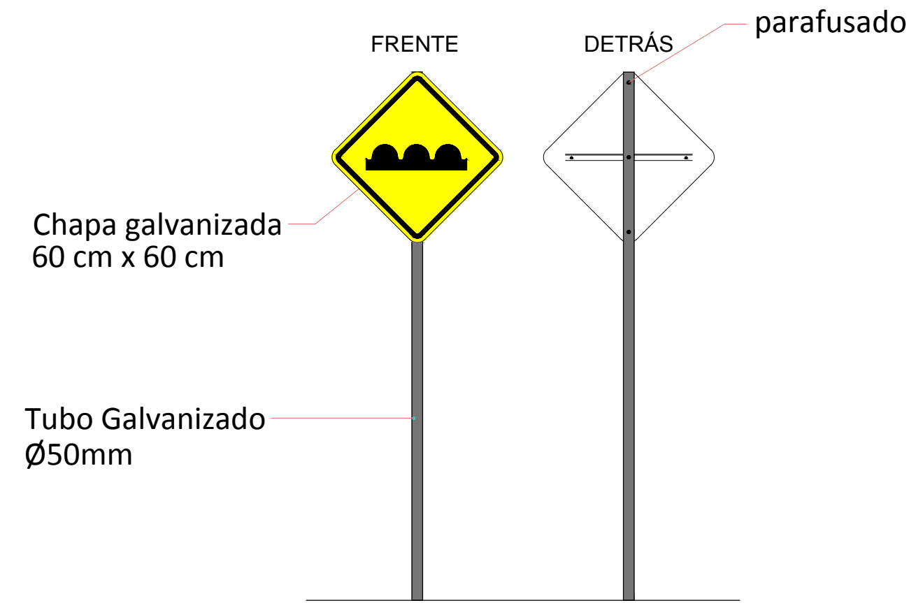
VISTA - PLACA SINALIZAÇÃO ESC: 1/25
